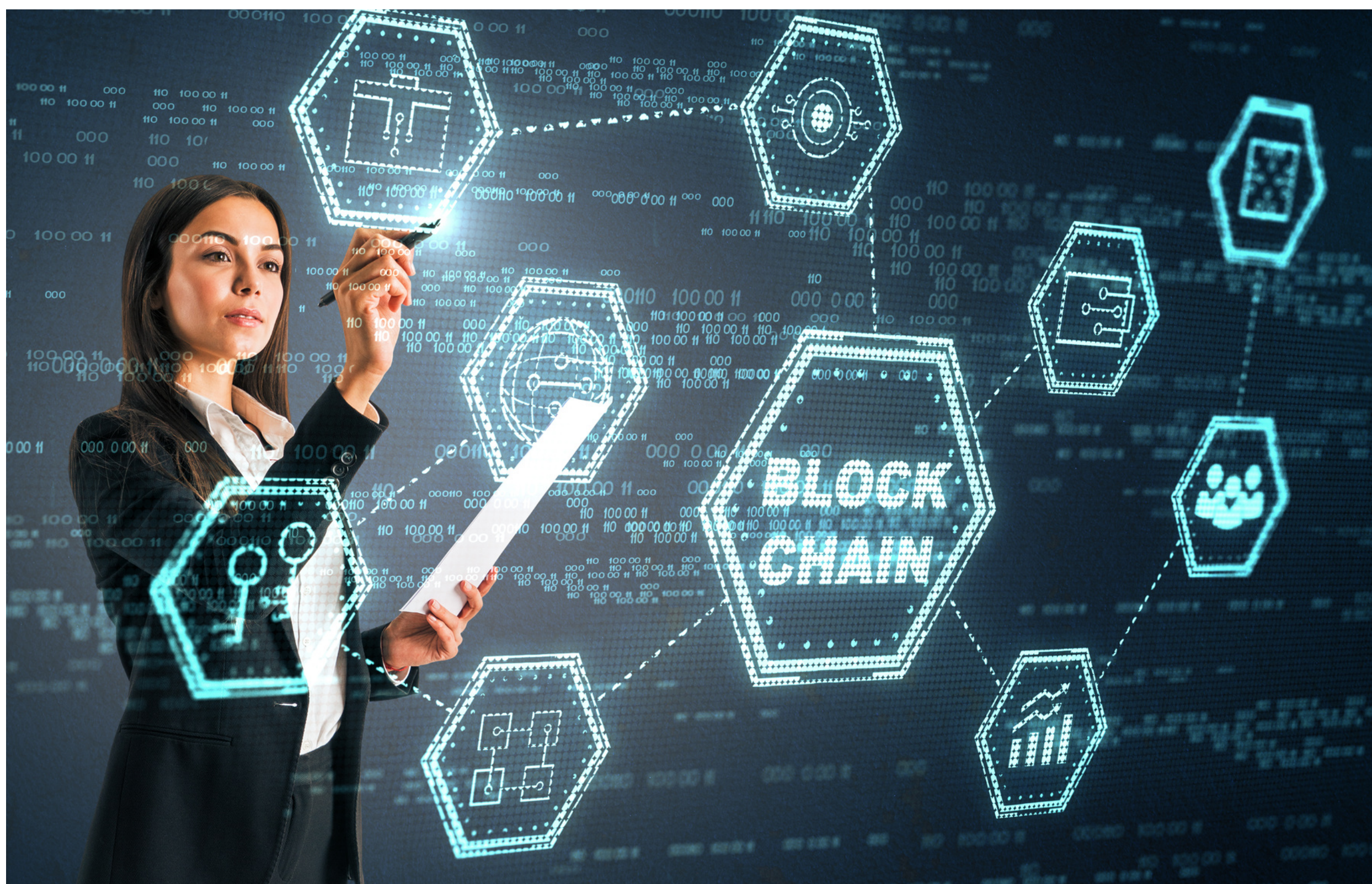
FIG. 3 - BLOCKCHAIN
